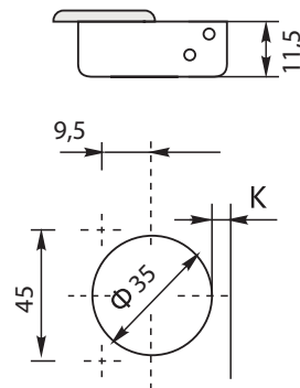
MDF ovi valk. Rondo2 saranaporaus
