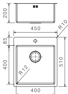
Upotusaukko 435 x 495 mm
