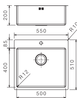
Upotusaukko 535 x 495 mm
