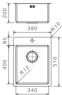
Upotusaukko 375 x 495 mm
